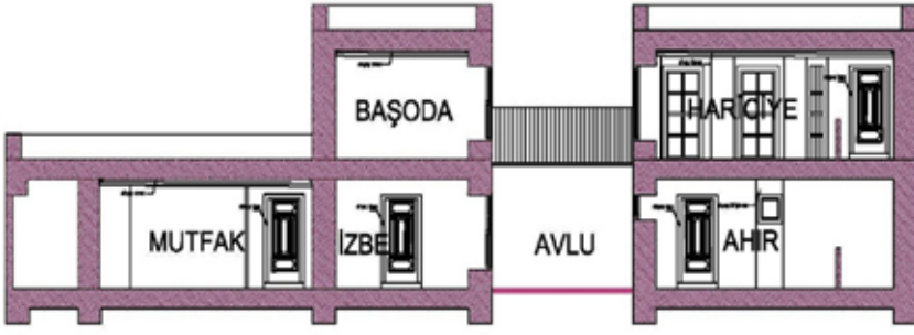
A - A KESİTİ
