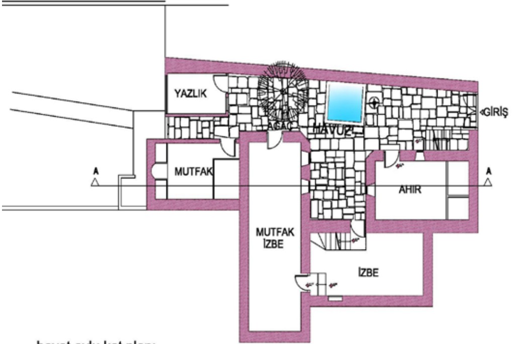
hayat avlu kat planı
