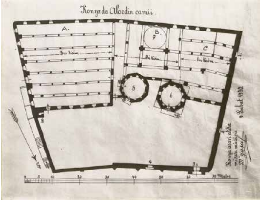
Alaaddin Camii planı
